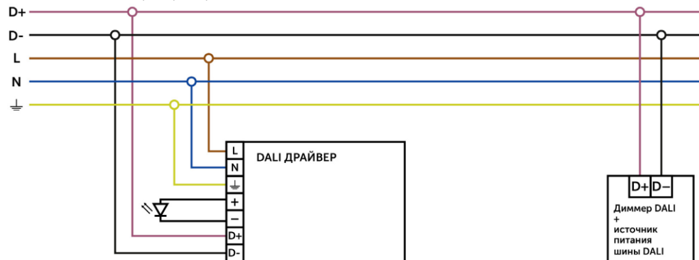
Схема подключения для драйверов серии LT20W DALI:
