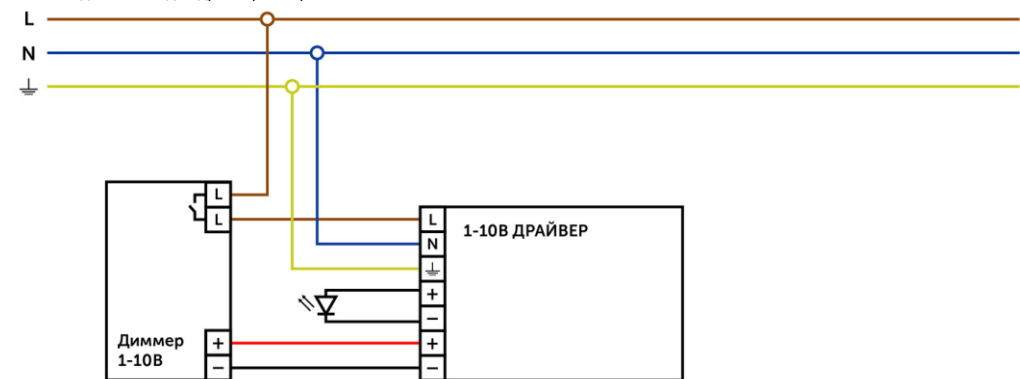
Схема подключения для драйверов серии LT20W 1-10V:
