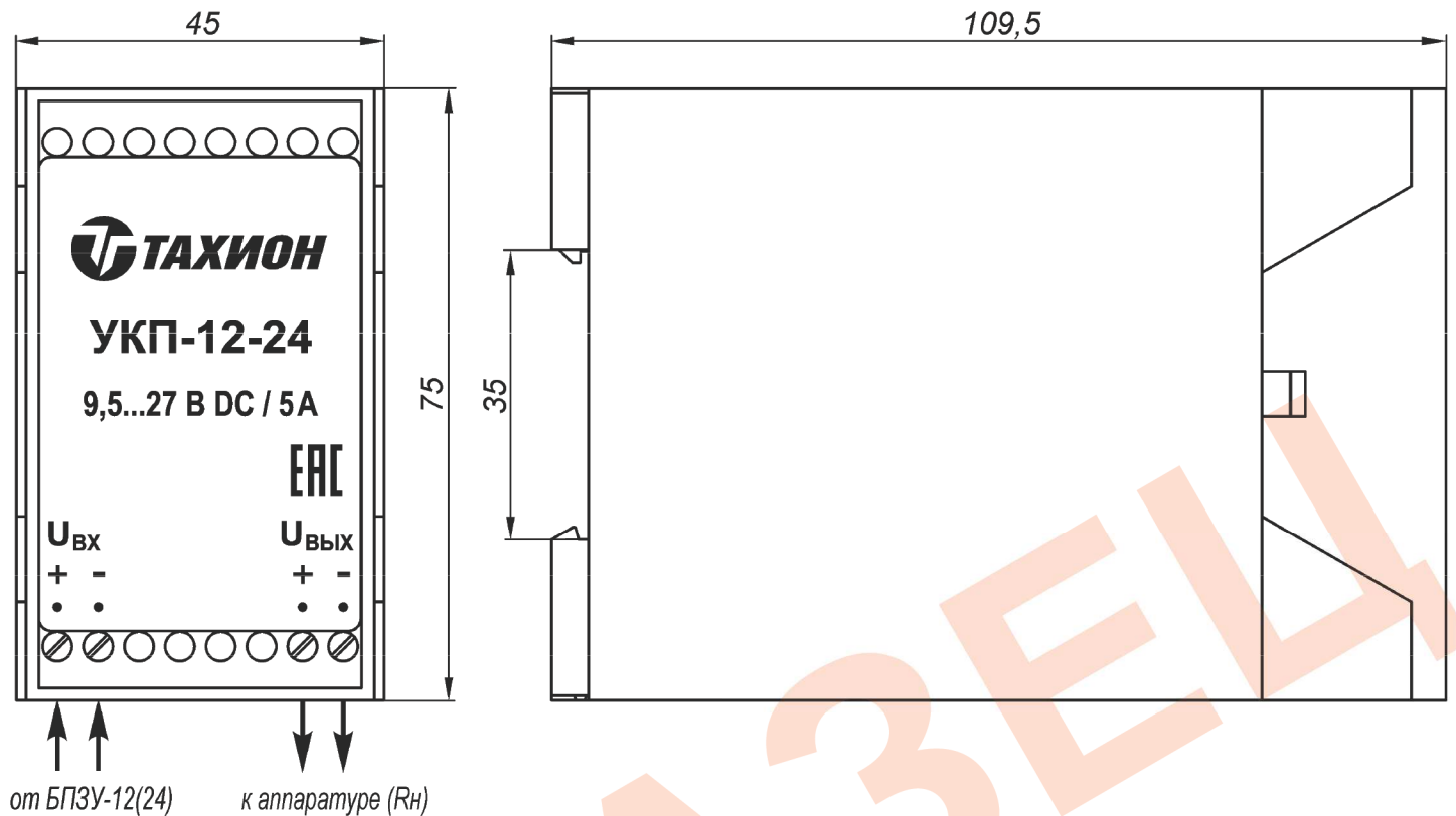
Рис.1 Схема подключения и габаритные размеры УКП-12-24
