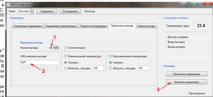
Рисунок 5. Режимы работы выхода OUT. Режим Сигнализация.
