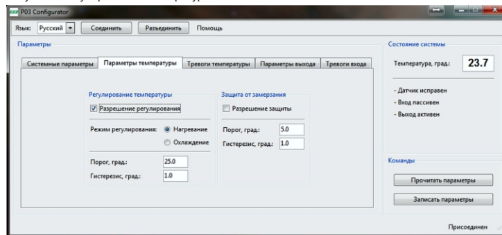
Рисунок 2. Регулирование температуры.
