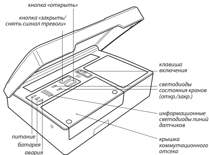
Рис. 2. Вид модуля управления Neptun ProW+ с открытой крышкой.
