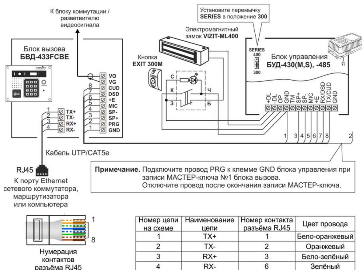
Рисунок 8.1 – Схема соединений блока вызова БВД-433ФСВЕ с блоком управления БУД-430(М,С), -485, электромагнитным замком VIZIT-ML400 и кнопкой EXIT 300M
