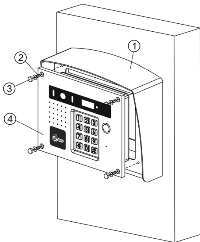
Рисунок 6.4 - Установка блока на монтажный комплект МКФ-432
