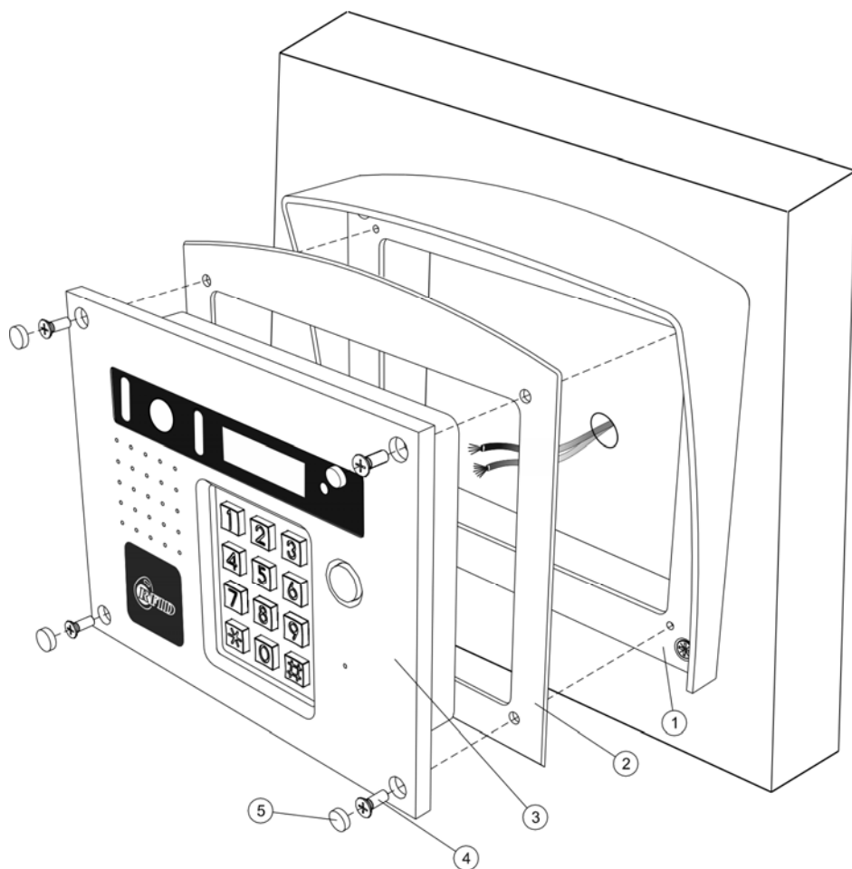
Рисунок 6.3 - Установка блока вызова на монтажный комплект МК-432
