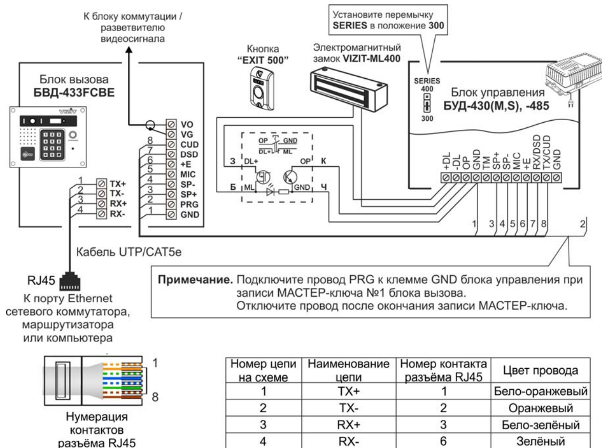
Рисунок 8.2 – Схема соединений блока вызова БВД-433ФСВЕ с блоком управления БУД-430(М,С), -485, электромагнитным замком VIZIT-ML400 и кнопкой EXIT 500
