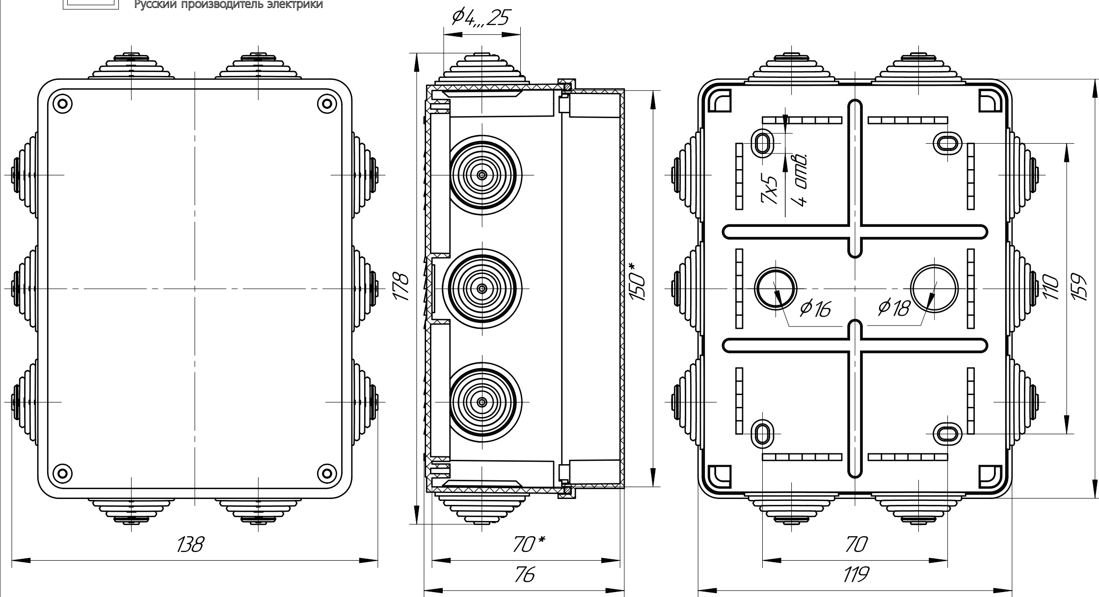
Чертеж 7: Коробка распределительная 40-0310 для о/п безгалогенная (HF) 150x110x70* Промрукав
