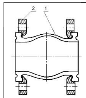
Рис. 7. Устройство типа ZKB. 1 – Гибкий элемент из армированной резины (EPDM или NBR); 2 – Фланец (2 шт.)
