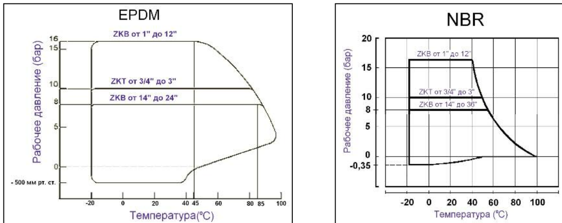
Рис. 5. Зависимость максимального рабочего давления от температуры перемещаемой среды для гибких вставок различных типов и диаметров.
