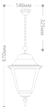
Схема НСУ-04-60-001
