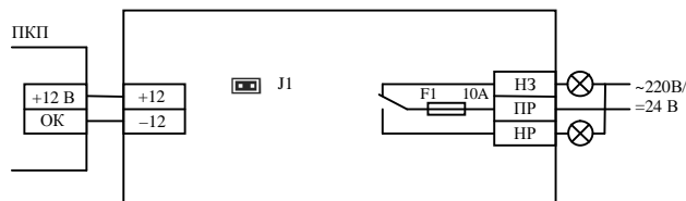
Рис. 2 Схема подключения БРВ к выходу приемно-контрольного прибора (ПКП) с ОК, цепь контроля СЛ подключена
