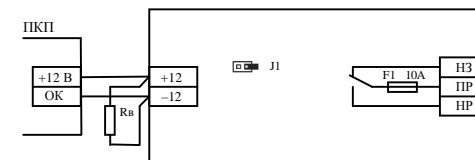
Рис. 4 Схема подключения БРВ к выходу ПКП с ОК, цепь контроля СЛ подключена, оконечный резистор отключен от 7,5 кОм
