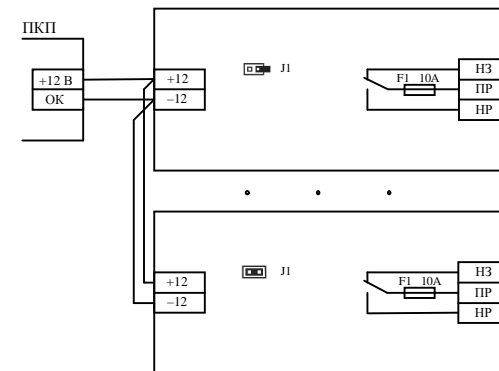
Рис. 5 Схема подключения нескольких БРВ к выходу ПКП с ОК, контроль СЛ до последнего БРВ
