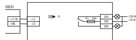
Рис. 3 Схема подключения БРВ к выходу приемно-контрольного прибора с ОК, цепь контроля СЛ отключена
