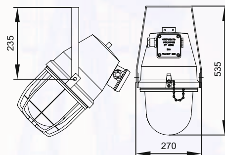
Размеры поворотного подвеса
