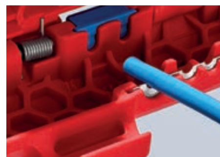
Практичный вспомогательный ограничитель облегчает ввод отдельных проводов для удаления изоляции
