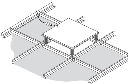
Рис. 1. Монтаж светильника в подвесной потолок типа «Армстронг» (модели PPL 595/R, PPL 595/U)
