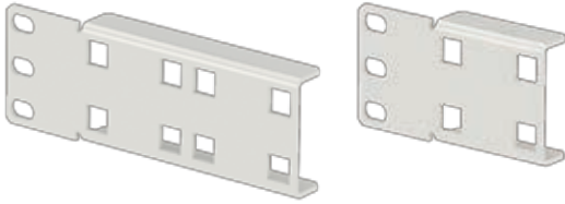
Кронштейн LZ короткий и длинный
