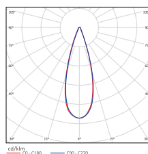
Угол излучения 30°
