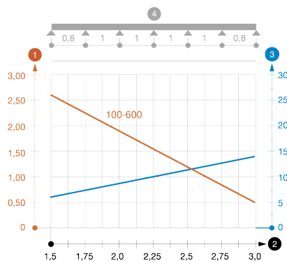
Диаграмма нагрузки
