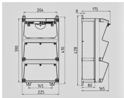
Чертеж 1 MB 522
