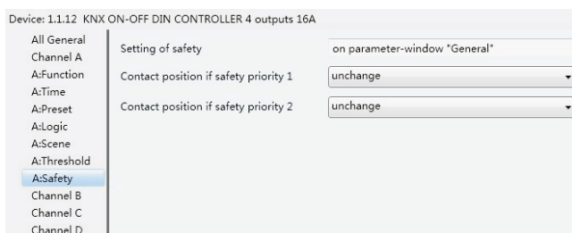
Рисунок 2.13. Окно настройки «X: Safety»
