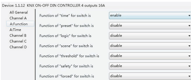
Рисунок 2.5. Окно настройки «X: Function»
