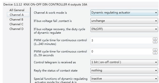
Рисунок 2.15. Окно настройки «channel: X-Dynamic regulating Actuator»
