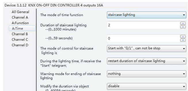
Рисунок 2.7. Окно параметров «X: Time-Staircase lighting» (X: время – лестничное освещение)
