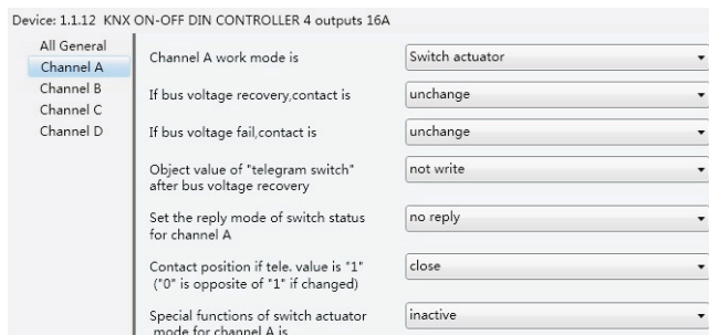
Рисунок 2.3. Окно параметров «Channel: X»
