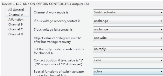
Рисунок 2.4. Вызов окна настройки «X: Function»
