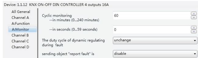
Рисунок 2.17. Окно параметров «X: Monitoring»
