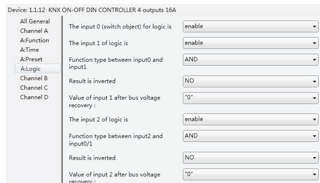
Рисунок 2.10. Окно настройки «X: Logic»
