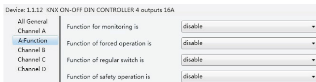
Рисунок 2.16. Окно настройки «X: Function»
