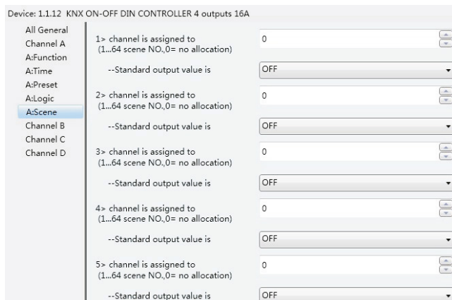
Рисунок 2.11. Окно параметров «X: Scene»
