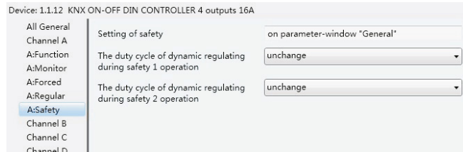
Рисунок 2.20. Окно параметров «X: Safety»
