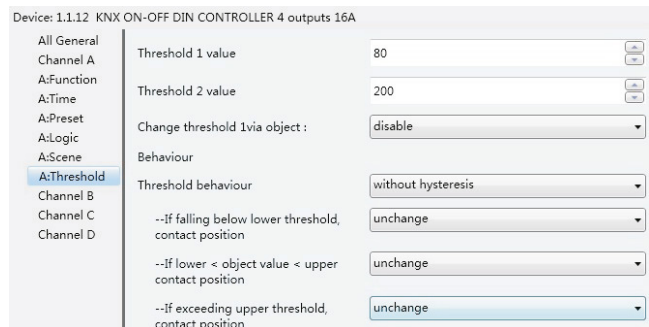
Рисунок 2.12. Окно настройки «X: Threshold»
