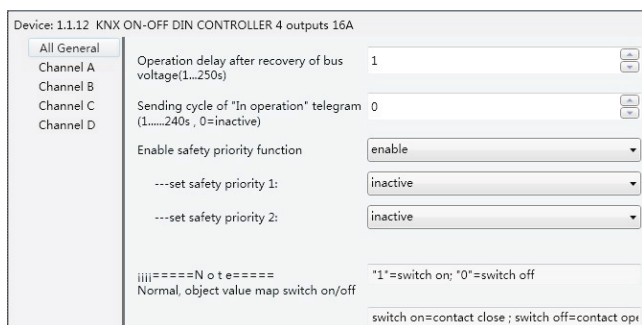
Рисунок 2.1. Окно параметров «All General»
