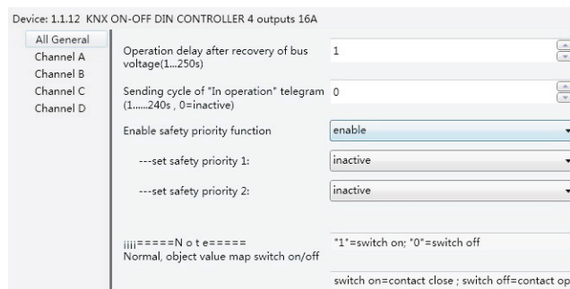
Рисунок 2.2. Окно параметра «Safety priority»
