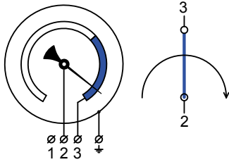
Исполнение I OP (один размыкающий контакт)
