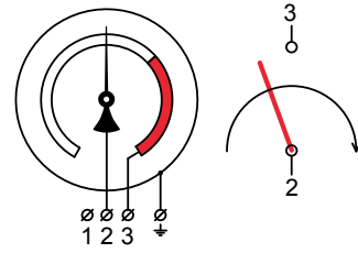
Исполнение I OЗ (один замыкающий контакт)
