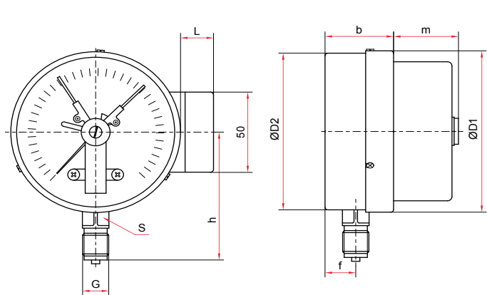
Радиальное присоединение
