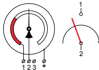
Исполнение II OЗ (один замыкающий контакт)
