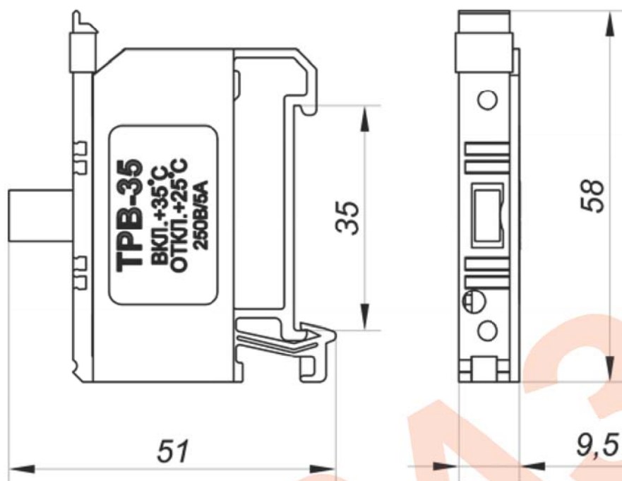
Рис.1 Габаритные размеры
