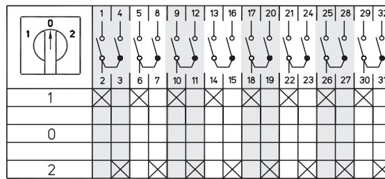
8-полюсные Схема 79
