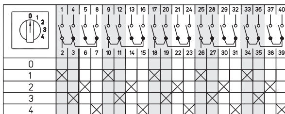
Схема 153
