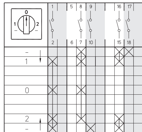
Тумблер с функцией хода влево или вправо Схема 210
