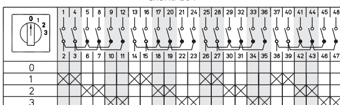
Схема 164
