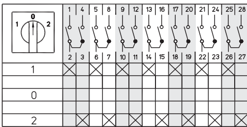
7-полюсные Схема 78
