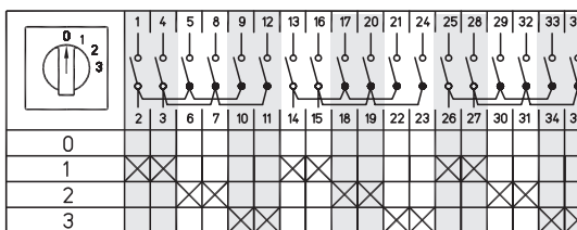
Схема 157
