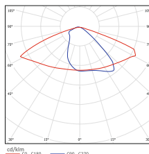
Угол излучения 150°x70°
