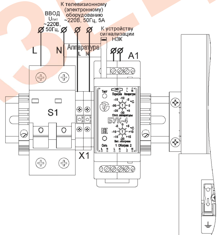
Рис. 2. Подключение термощафа
