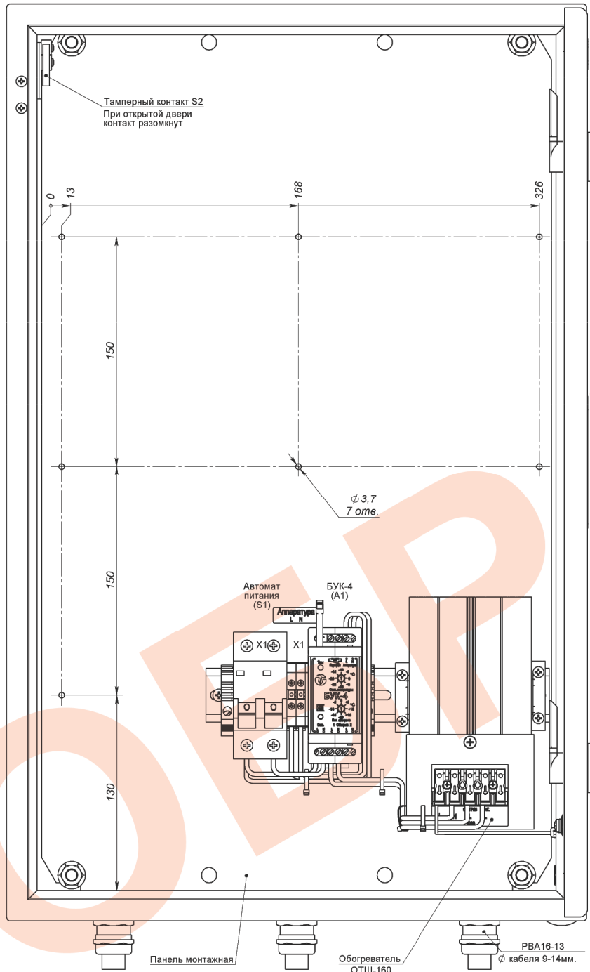
Рис.1. Устройство термощафа (дверь открыта на 90°)
