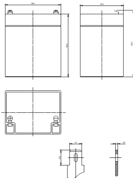
Вывод Ш-6,35
