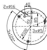
Схемы установки светильника:
