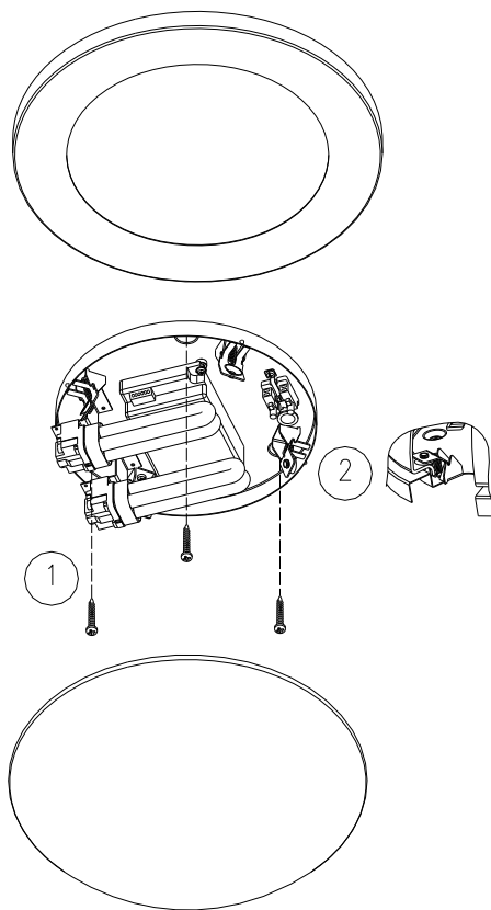
Схемы установки светильника:
