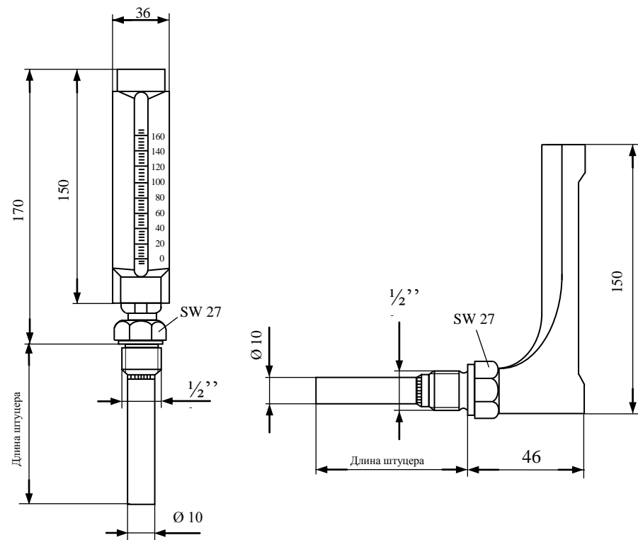
Термометр MTG
