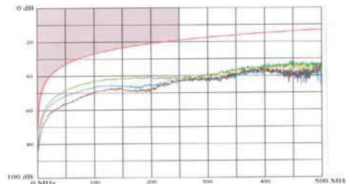
Примерный график измерения PS ELFEXT кабеля F/UTP категории 6 производства КЗ MADEX
