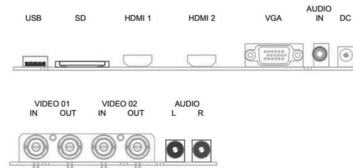
Рис. 1 Схема расположения и назначение разъемов.
