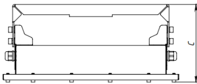
Габаритные размеры светового указателя (для установки в проем), мм
