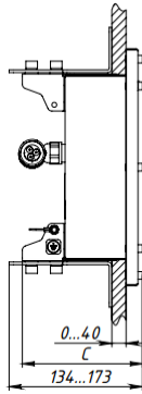
Габаритные размеры светового указателя (для установки на стену), мм
