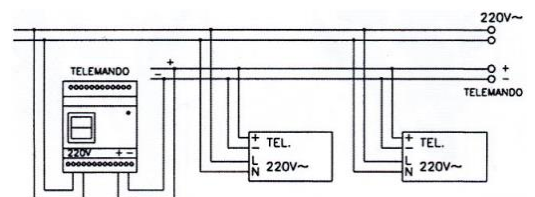
Схема подключения светильников с Telemando
