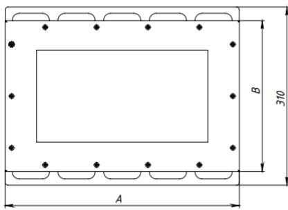
Габаритные размеры светового указателя (для установки в проем), мм
