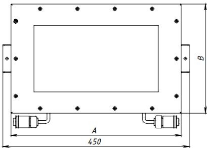
Габаритные размеры светового указателя (для установки на стену), мм
