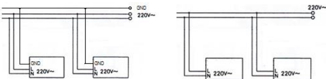
Схема подключения светильников для централизованных систем питания
