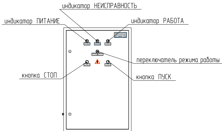
Рисунок 2 - Внешний вид ШУН
