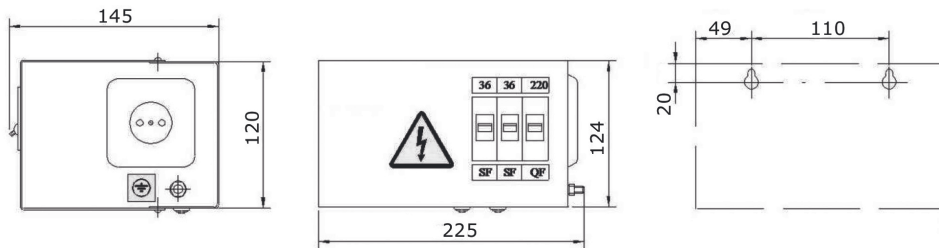
Рисунок А.1. Ящик ЯТП-0,25-220-IP31-УХЛ3, масса не более 5 кг
