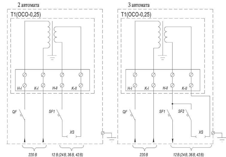
Рисунок А.2. Схема электрическая принципиальная ЯТП-0,25-220УХЛ3 IP-31
