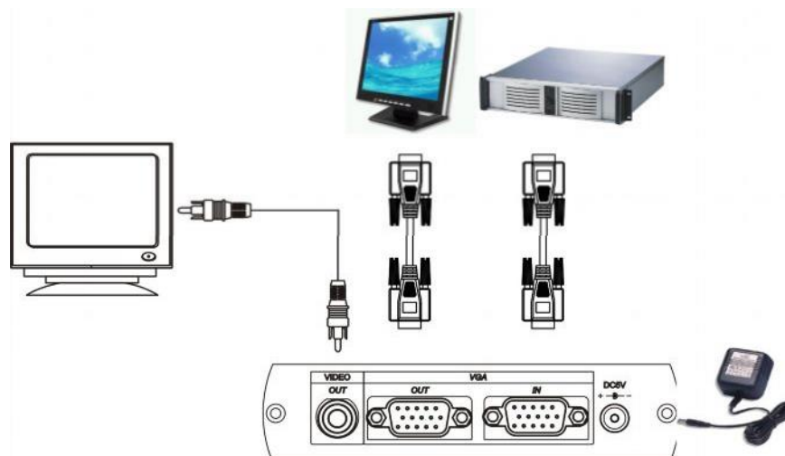
Рис.2 Структурная схема подключения
