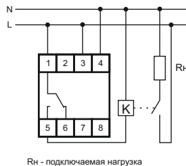
Схема подключения изделия с использованием контактора ток нагрузки более 16А.
