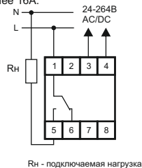
Схема подключения изделия и нагрузки, питающихся от разных источников питания.
