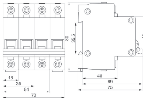
Рисунок В.1 Габаритные, установочные, присоединительные размеры выключателей.
