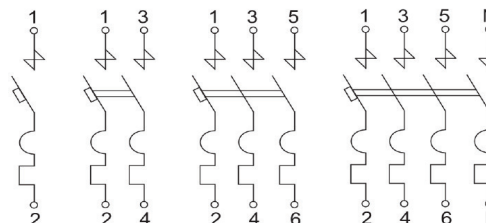
Рисунок Г.1 Принципиальные электрические схемы выключателей
