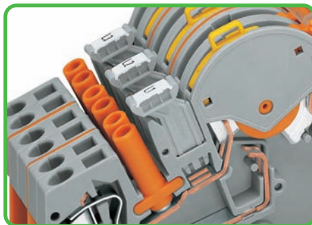
Держатели групповой маркировки позволяют маркировать подгруппы в ограниченном пространстве. Они могут быть установлены в разъемы для перемычек в клеммах. Маркировочная система: маркеры WMB
