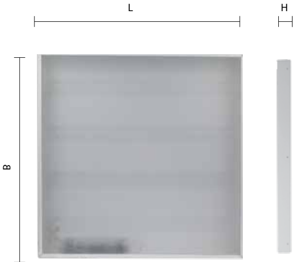
* Корпус светильника потолочного исполнения
