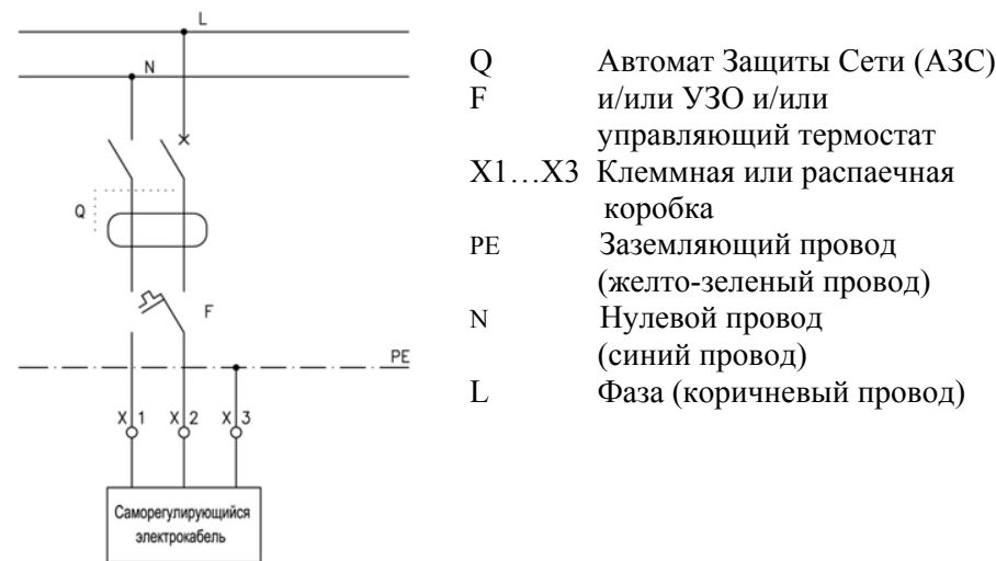
Рис. 5. Схема подключения электрообогрева кровельной воронки HL62.1H к электрической сети.
