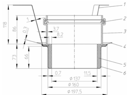
Рис. 7. Противопожарная муфта HL870 для кровельной воронки HL62.1H/1.
