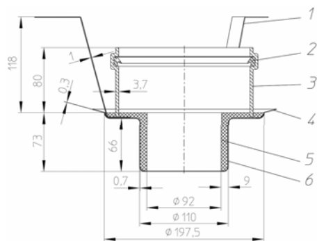
Рис. 6. Противопожарная муфта HL850 для кровельной воронки HL62.1H/7.
