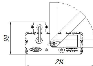
Светильник ПС 2 с креплением скоба
