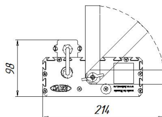
Светильник ПС 3 с креплением скоба
