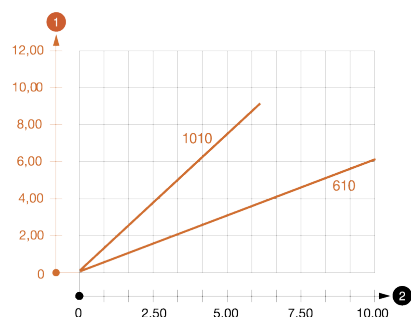
Диаграмма нагрузки
