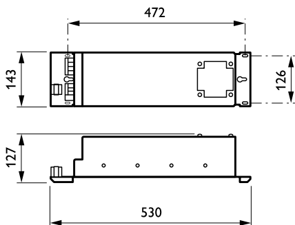
GearUnits ECM330/ECF330
