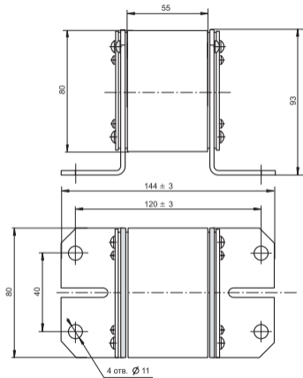
Рисунок Б.6.а) Исполнение ПП60С-41Т - уголковое на 1000 А
