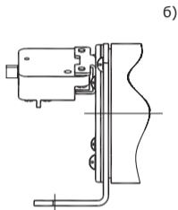
Типоисполнение с указателем срабатывания и свободным контактом, расположенным под углом
