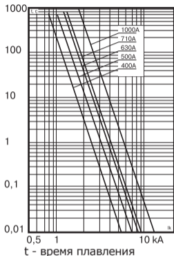
Рисунок В.3. Преддуговые время-токовые характеристики
