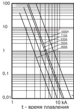
Рисунок В.4. Время-токовые характеристики отключения при напряжении 730 В
