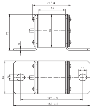
Рисунок Б.3. Исполнение ПП60С-(37,38,39,40)У - угловое с одним отверстием
