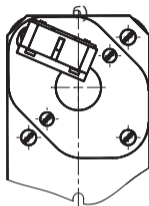
Типоисполнение с указателем срабатывания и свободным контактом, расположенным под углом
