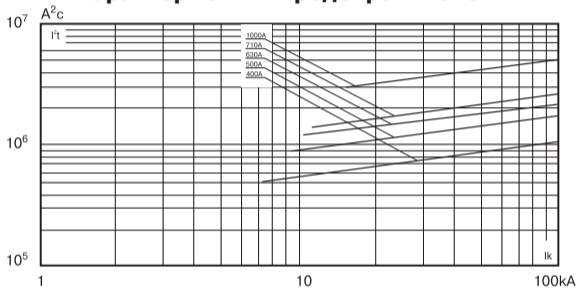
Рисунок В.1. Характеристики интеграла Джоуля отключения при напряжении 730 В
