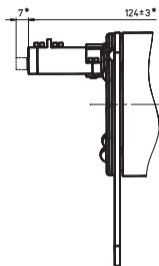
Типоисполнение с указателем срабатывания и свободным контактом
