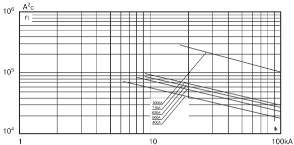
Рисунок В.5. Характеристики преддугового интеграла Джоуля
