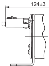
Типоисполнение с указателем срабатывания и свободным контактом
