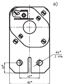
Рисунок Б.8.а) Исполнение ПП60С-41КП - (консольное с пря- мым верхним выводом) на 1000 А
