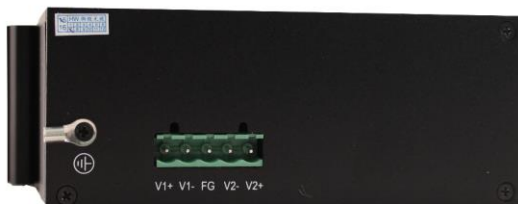
Рис.2 Коммутатор SW-60802/IC, вид спереди/сбоку
