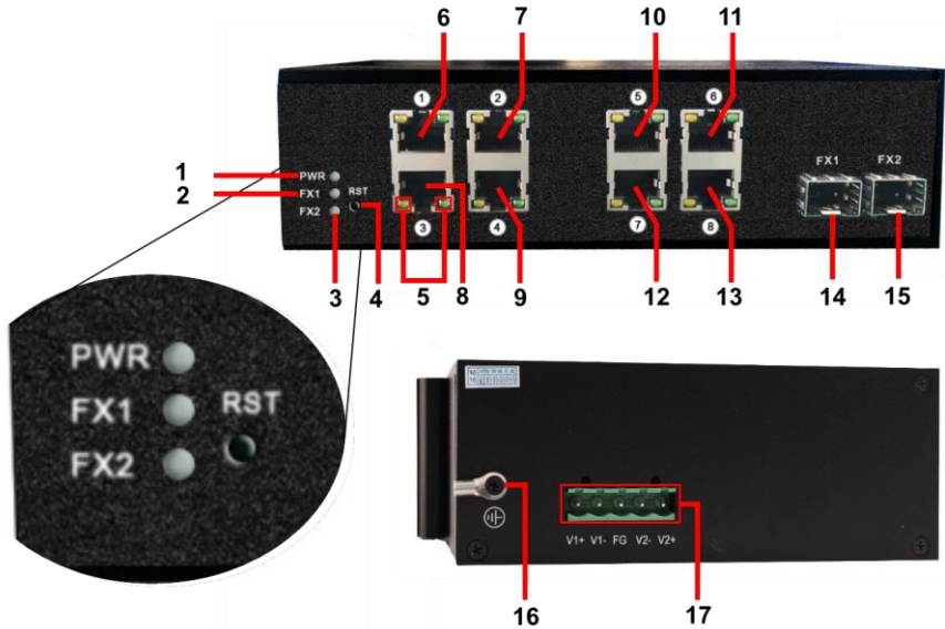
Рис. 3 Разъемы, кнопки и индикаторы коммутатора SW-60802/IC
