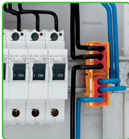
Подключение одножильных и многожильных проводников 6 мм²/AWG 10.
