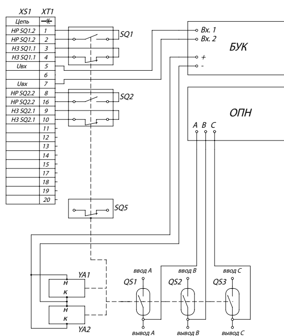
Схема электрическая принципиальная контакторов на 36, 110 В
