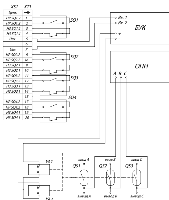
Схема электрическая принципиальная контакторов на 220, 380 В
