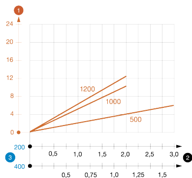
Диаграмма нагрузки
