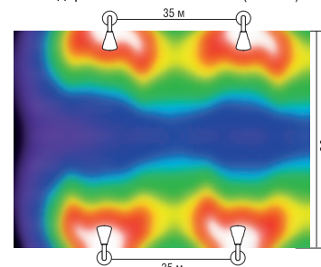
Стандартный светильник ГКУ (400 Вт)
