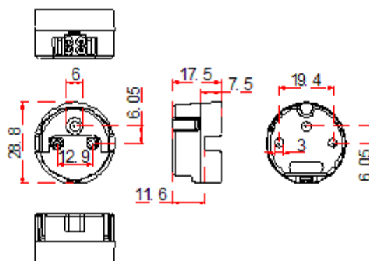
Патрон (ламподержатель) G13 накладной для люминесцентных ламп T8, T12 (крепление - винт)
