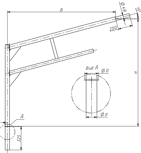
Кронштейны серии 2 под 2 консольных светильника однонаправленные на круглоконические и граненые опоры
