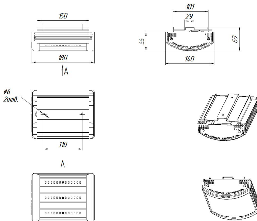
Светильник СПО 12; потолочное крепление
